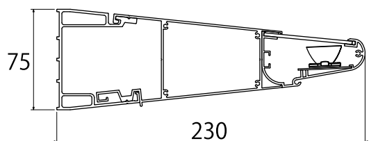
断面図
