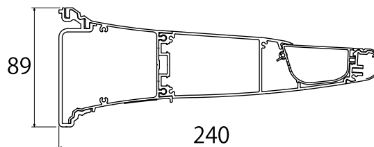
断面図
