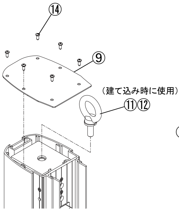
詳細図 A
