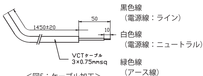
<図5：ケーブル加工>
