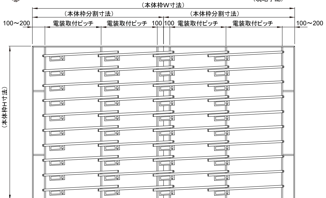
電装の配置例
