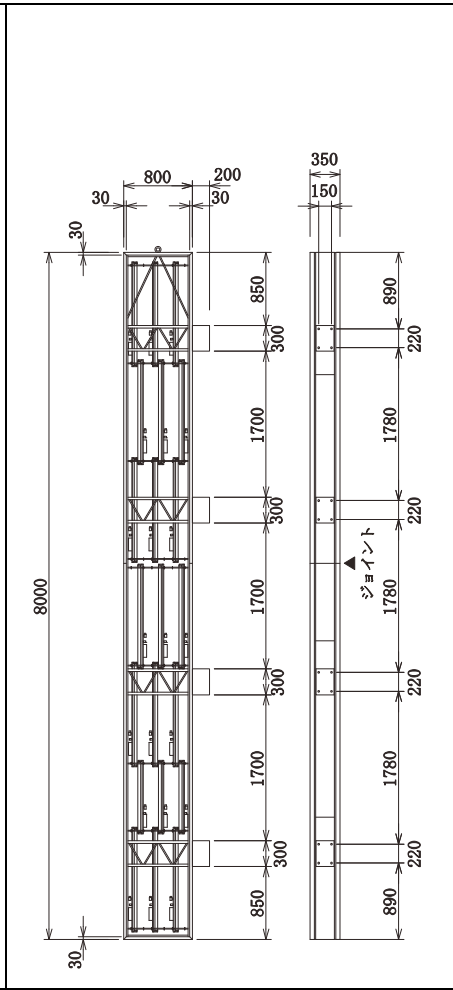
品番 FT0805 (品名 FF880) W800×H8000×D350
