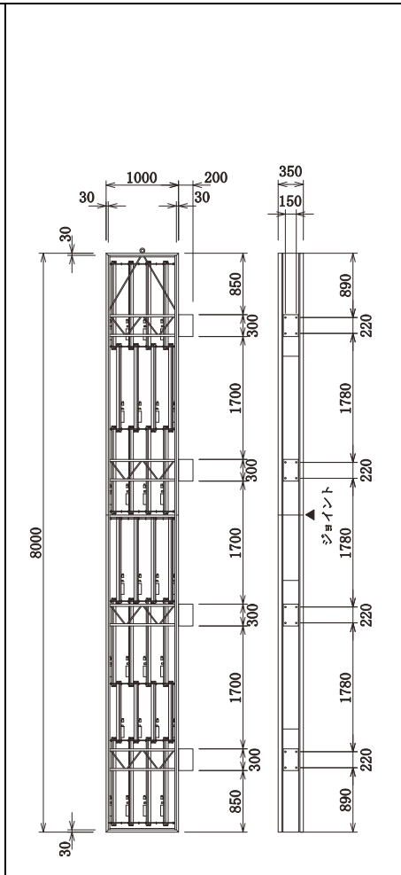
品番 FT1005 (品名 FF1080) W1000×H8000×D350
