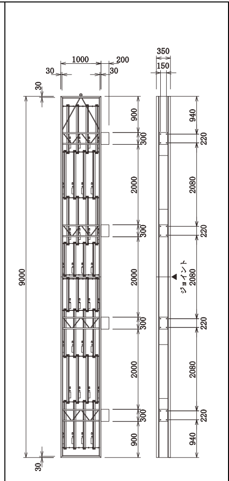
品番 FT1006 (品名 FF1090) W1000×H9000×D350
