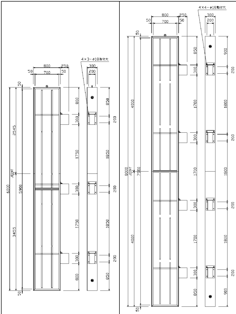
品番：69-69 品名：押縁 860
