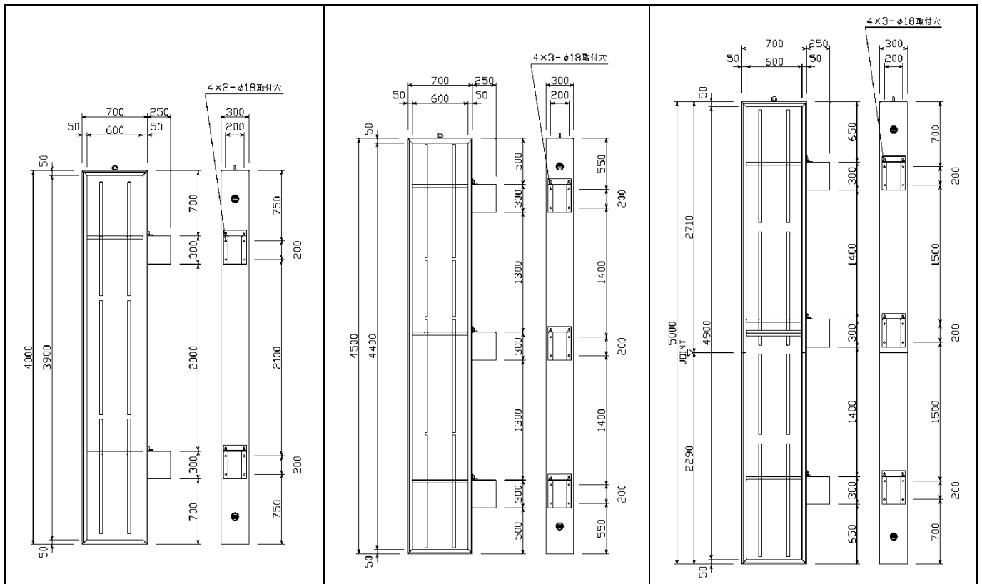
品番：69-61 品名：押縁 740
