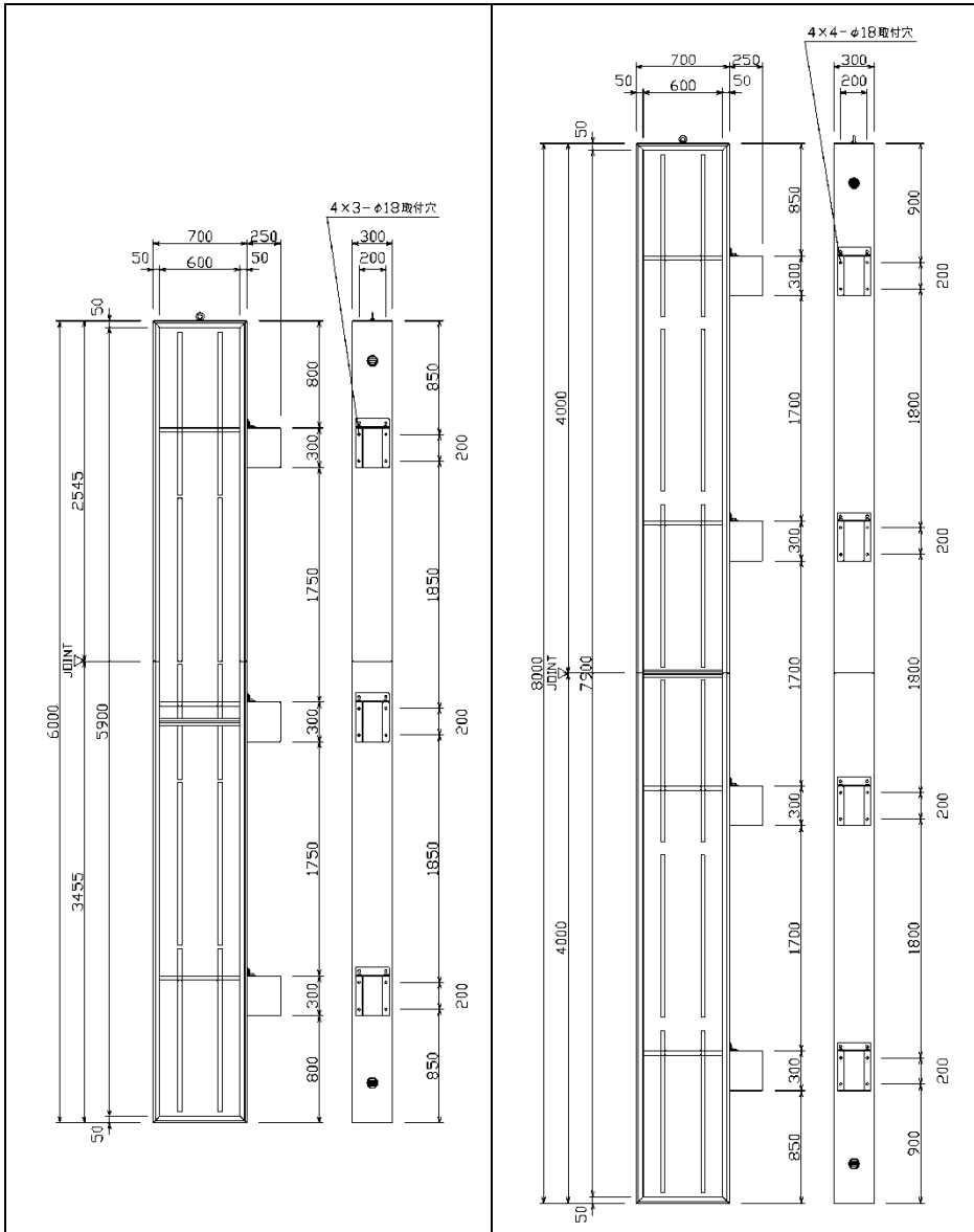
品番：69-64 品名：押縁 760
