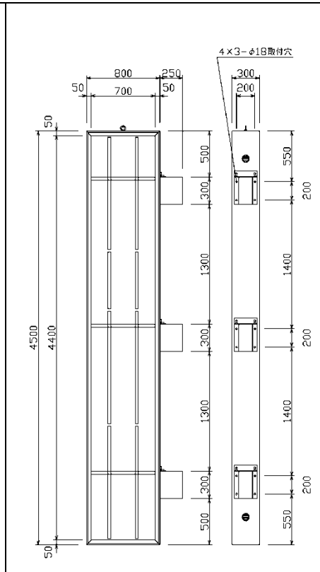
品番：69-67 品名：押縁 845
