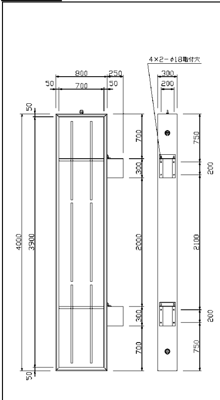
品番：69-66 品名：押縁 840
