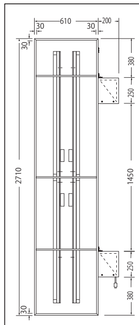
■足ピッチ 詳細図
